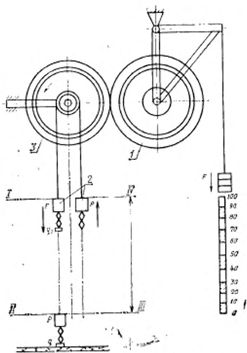
1—штанна на ободу; 2—грузы; 3—барабан
